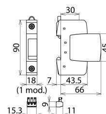
Dimension drawing DG SU 1P 240 R
