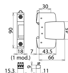
Dimension drawing DG SU 1P 347 R
