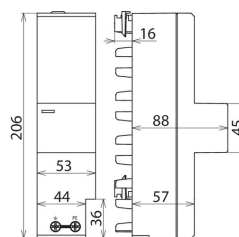
Dimensions DSH ZP TT 255
