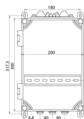
Dimension drawing IGA 10 V2 IP54
